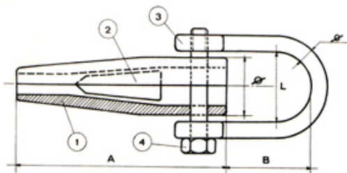
1 = CONE 2 = WEDGE 3 = SHACKLE 4 = T. PLUG
